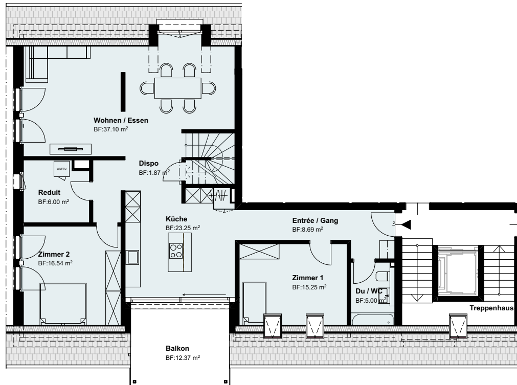
1. Dachgeschoss
